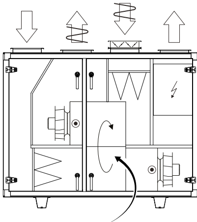
Warmtewisselaarrotor
