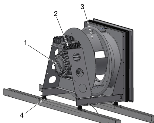
Ventilatorenhed størrelse 480-1540
